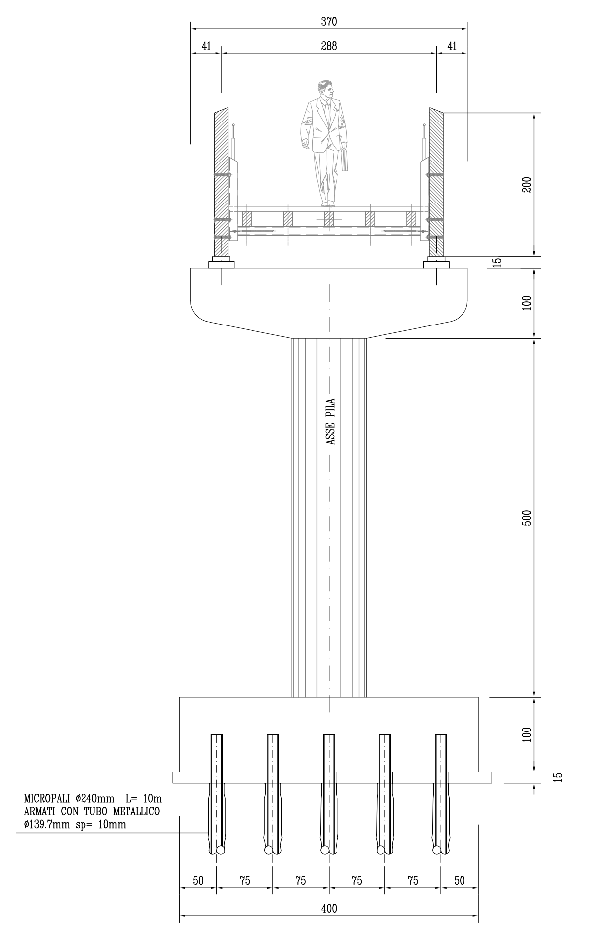
SEZIONE TRASVERSALE PILA CENTRALE scala 1:50
