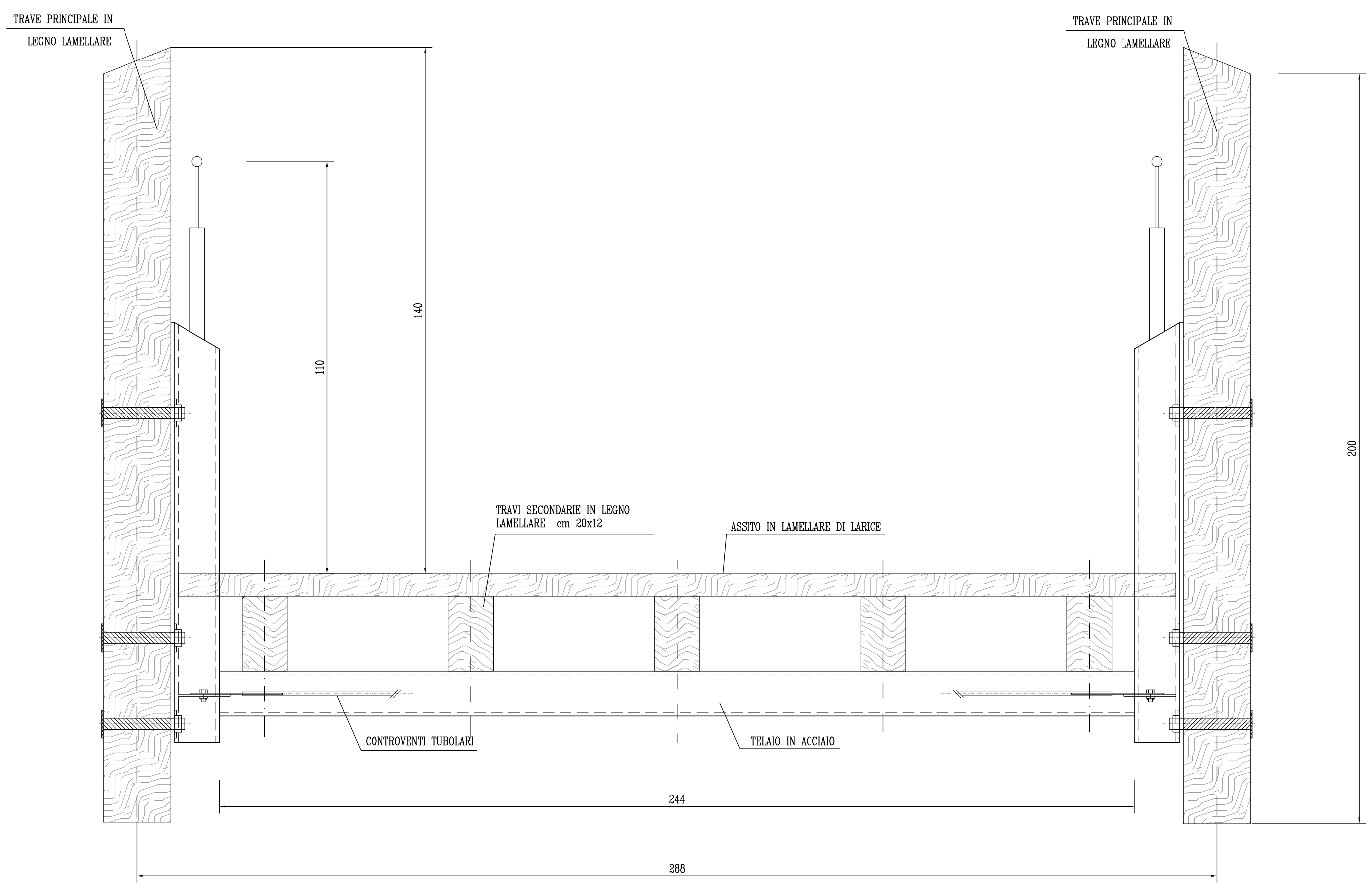
SEZIONE TRASVERSALE B-B scala 1:10
